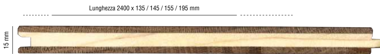
Sezione doga 1:1
